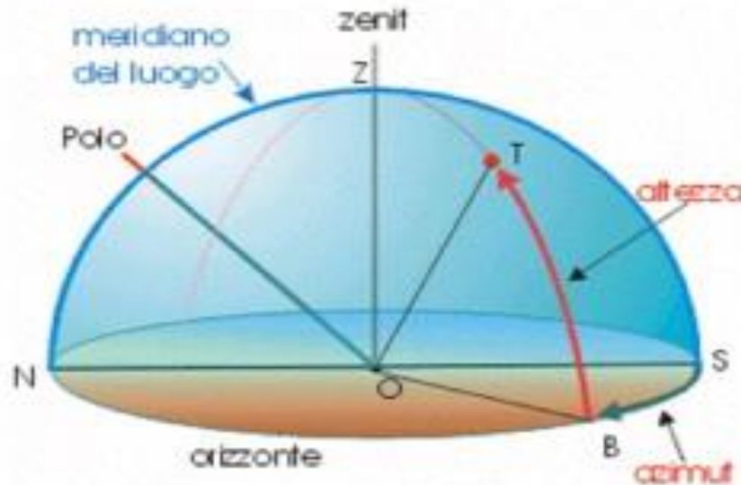
Coordinate altazimutali
